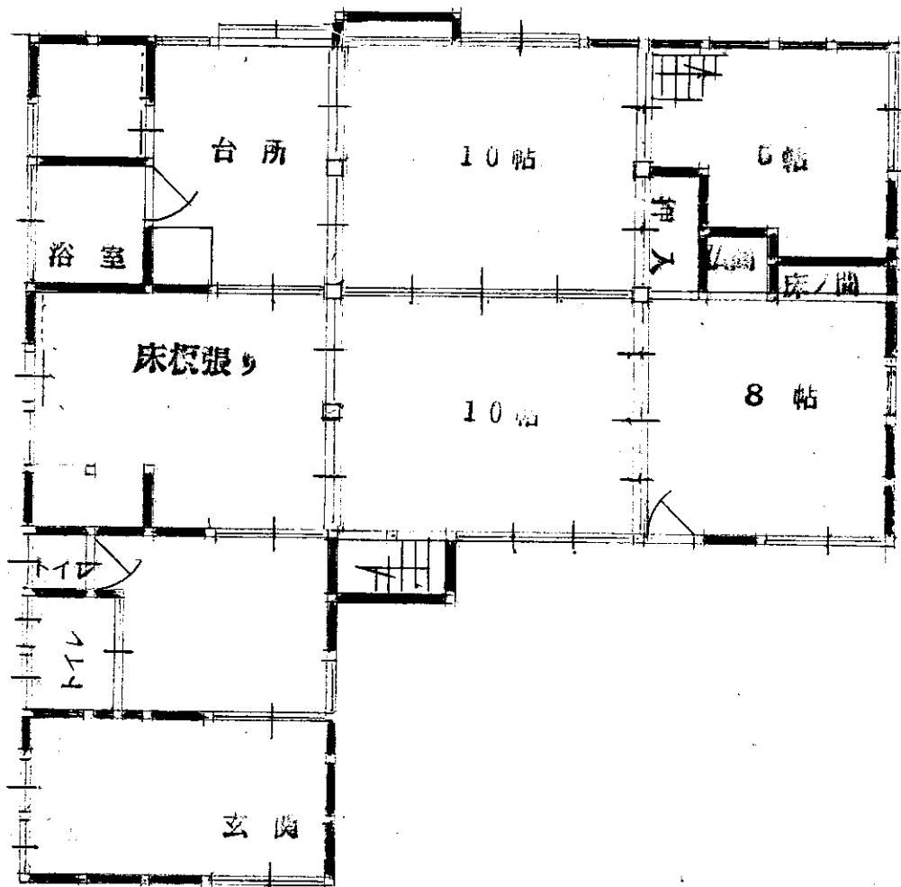
一階平面図 S=1/100 35.83 118.41
